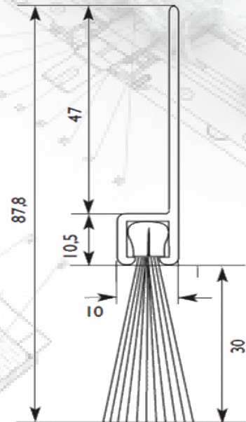
ELASTO-SEAL DXL (Nylon noir, \varnothing : 0,203 mm)
