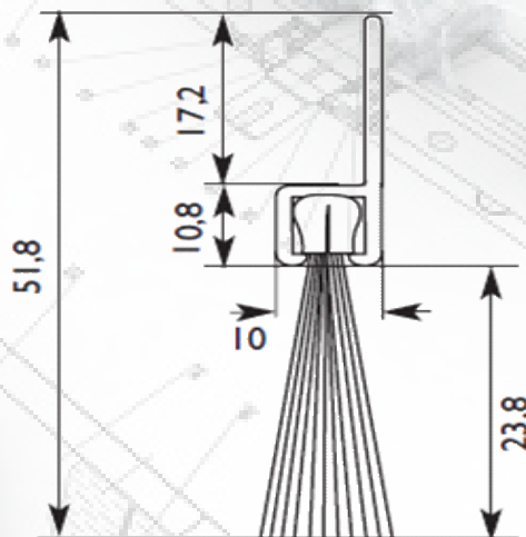
ELASTO-SEAL D (Nylon noir, \varnothing : 0,203 mm)
