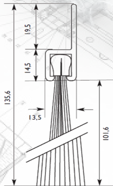
ELASTO-SEAL GL (Nylon noir, \varnothing : 0,508 mm)
