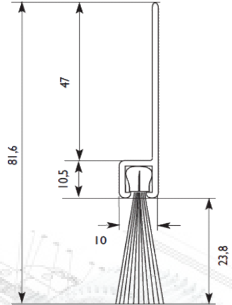
ELASTO-SEAL DL (Nylon noir, \varnothing : 0,203 mm)
