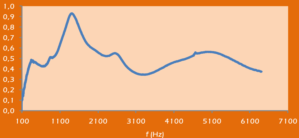
Coefficient d'Absorption
