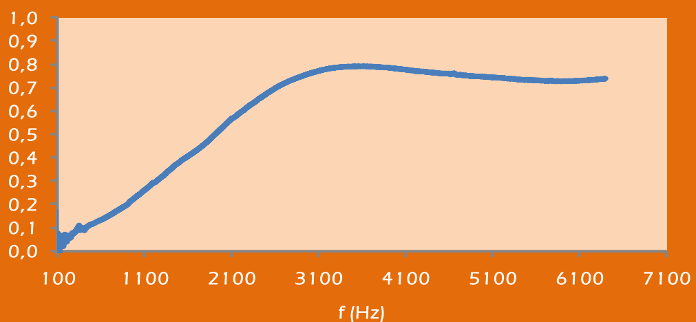
Coefficient d'Absorption
