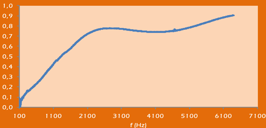
Coefficient d'Absorption
